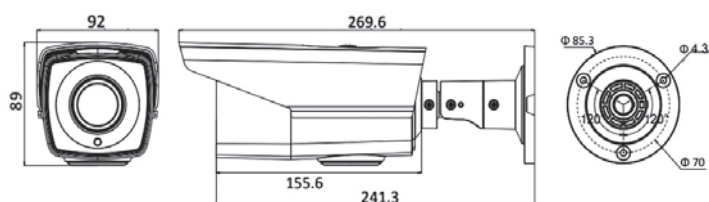
■寸法図 (Unit : mm)
